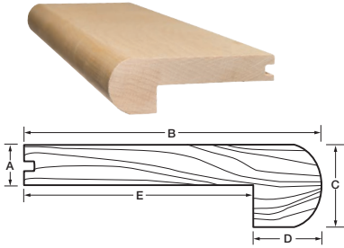
Nez de marche rond (Installation collée)
