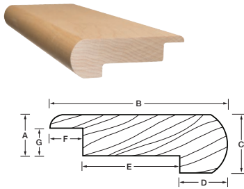
Nez de marche rond (Installation non fixée)
