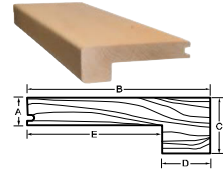
Nez de marche au rebord carré 1/2 po
