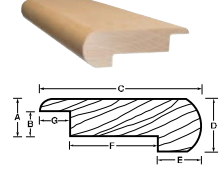
Nez de marche au rebord rond 7/16 po Pour installation non fixée
