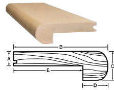
Nez de marche au rebord rond 1/2 po
