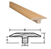
Mouleur en « T »
