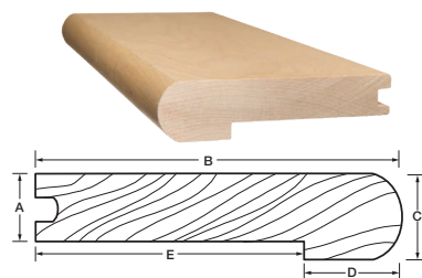
Nez de marche rond
