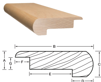
Nez de marche rond (Installation non fixée)
