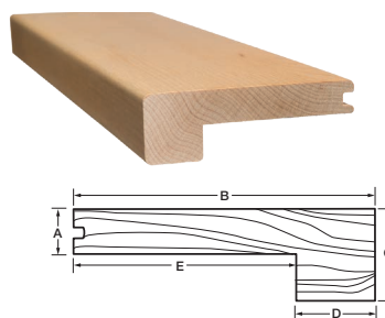
Nez de marche carré
