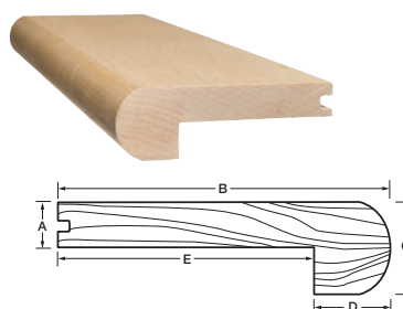
Nez de marche rond
