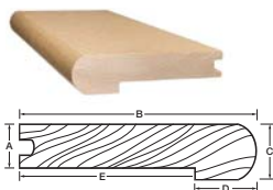
Nez de marche au rebord rond 3/4 po
