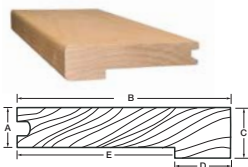
Nez de marche au rebord carré 3/4 po*
