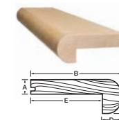
Nez de marche au rebord rond 3/8 po
