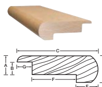
Nez de marche au rebord rond 7/16 po
