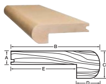
Nez de marche au rebord rond 1/2 po
